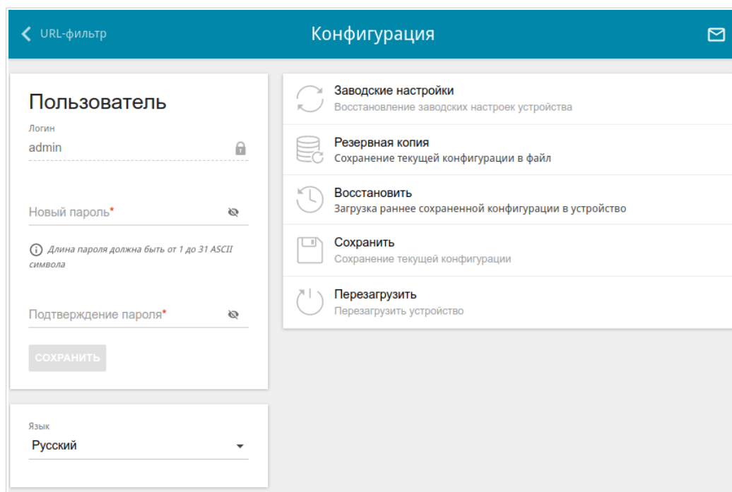
Рисунок 136. Страница Система / Конфигурация .
