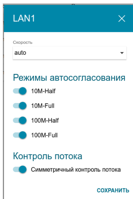
Рисунок 110. Окно изменения настроек порта маршрутизатора.
