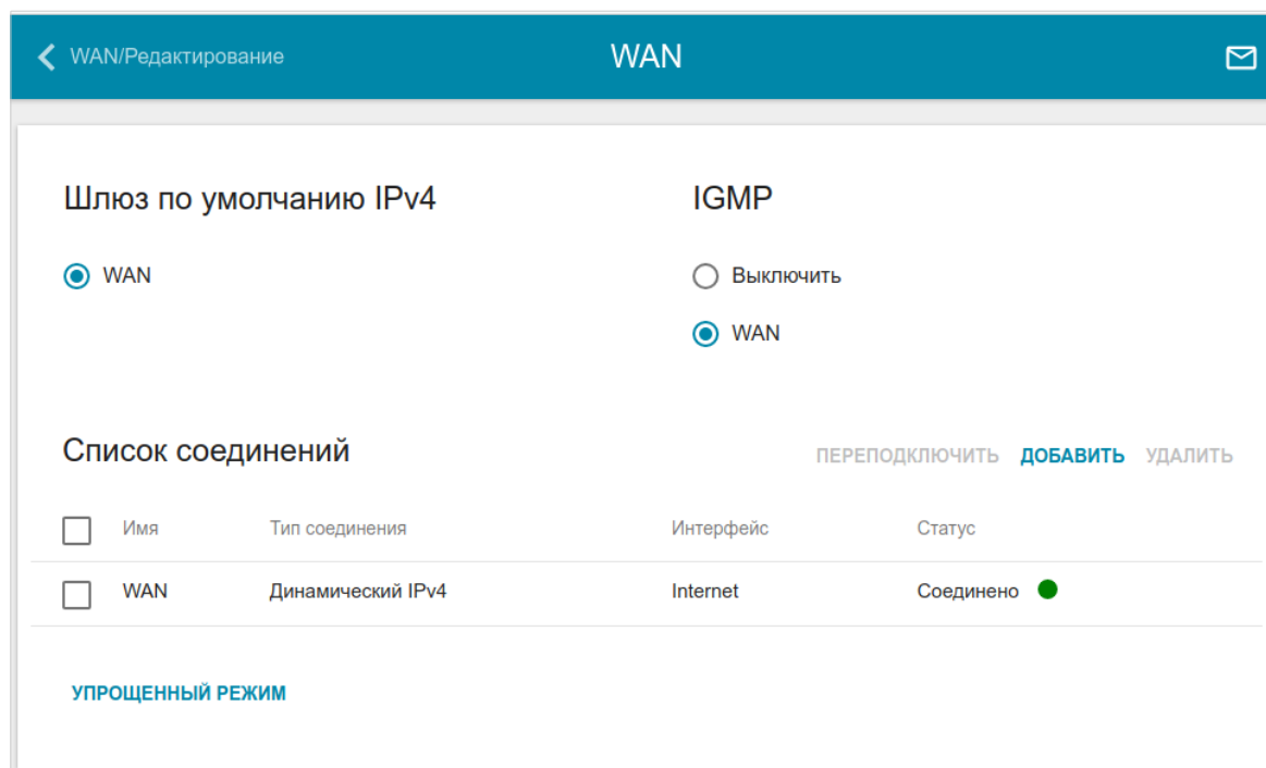
Рисунок 57. Страница Настройка соединений / WAN . Расширенный режим.
